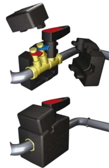
Клапан Venturi может быть установлен непосредственно за изгибом трубопровода.
